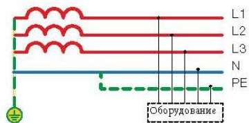
TNC-S 230 / 400 V
