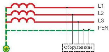
TNC 230 / 400 V
