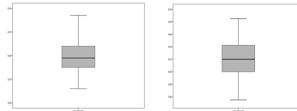
а. Поправка значимости Лильефорса
