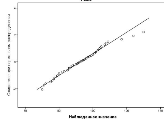
Вероятностный график (квантили) для Частота сердечных сокращений лежа
