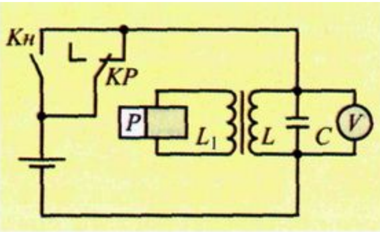
Мал. 3. 17. Схема електричного кола для одержання незатухаючих коливань з електромагнітним реле
