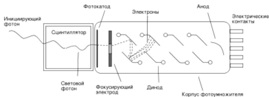
Схема ФЭУ
