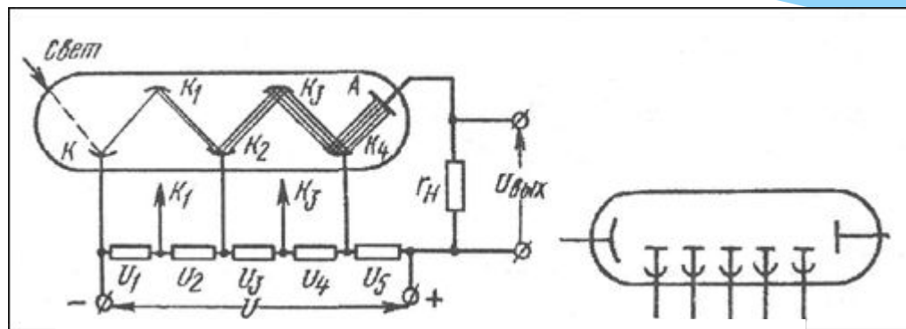
Схематичное изображение ФЭУ
