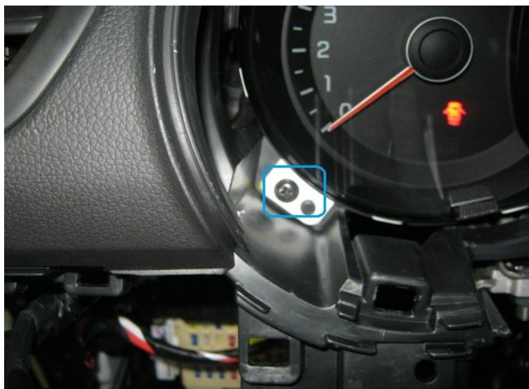
Фото 3.3. Крепление приборного щитка
