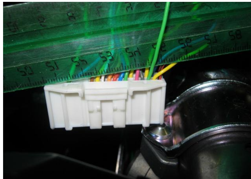
Фото 11.2. Концевик дверей (Зелёный, №3 разъёма M01-A)
