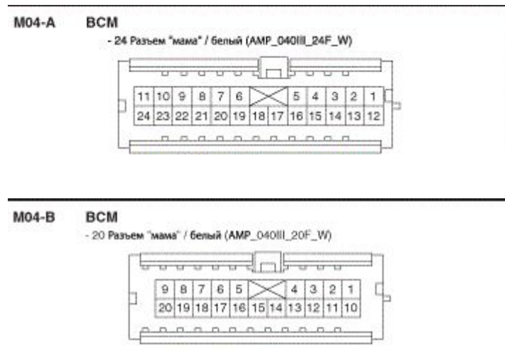
Фото 13.1. Разъёмы блока BCM
