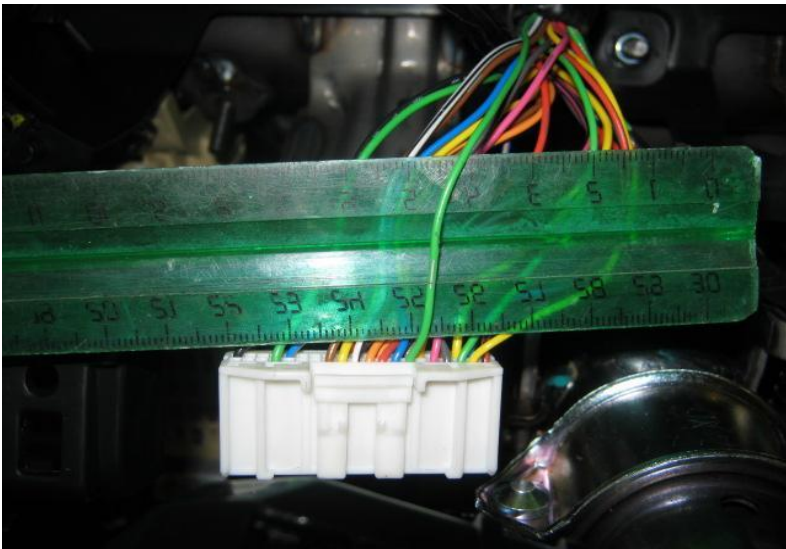
Фото 11.3. Концевик багажника (Зелёный, №7 разъёма M01-A)
