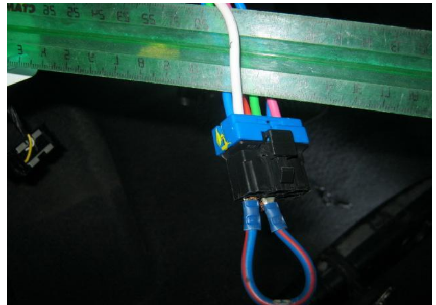
Фото 14.5. Стартер (Синий, № 4 разъёма M17)
