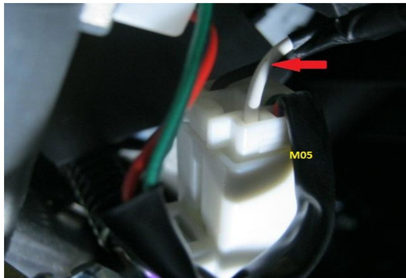
Фото 7. Я брал белый провод (№ 1 разъёма M05)
