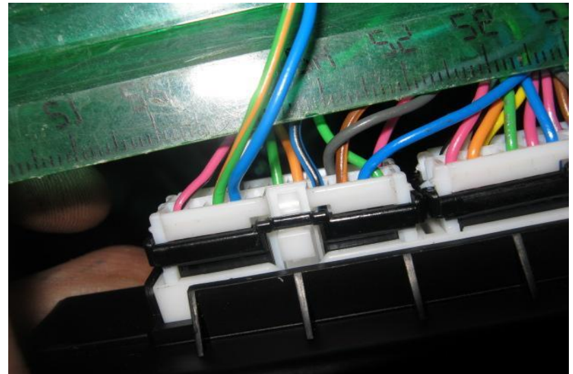
Фото 13.2. Управление Ц.З. (Синий/запирание, Зелёный с оранжевой полосой/отпирание), № 6 и № 7 разъёма M04-B)
