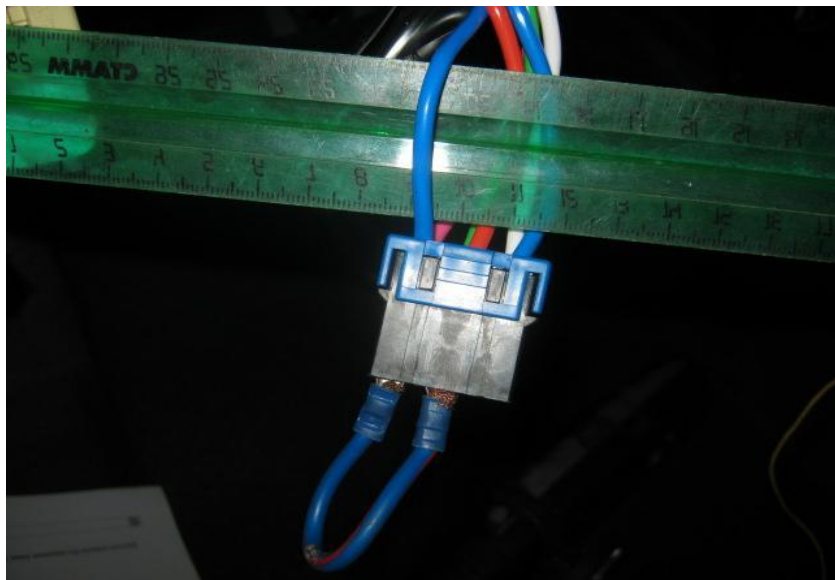
Фото 14.2. Зажигание 1 (Синий, № 4 разъёма M17)
