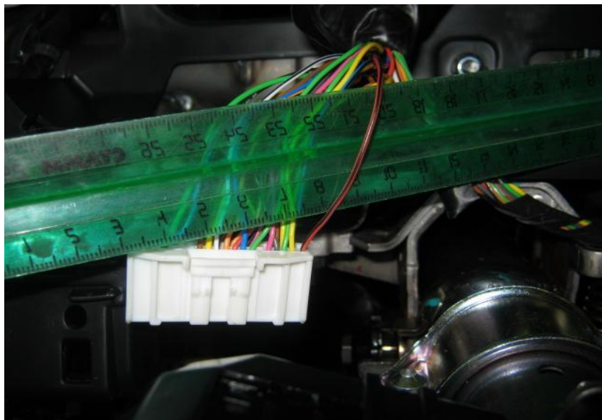
Фото 11.1. Ручник (Красный с чёрной полосой, № 1 разъёма M01-A) Только для МКПП
