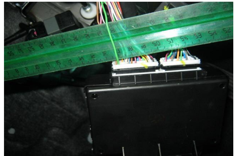
Фото 13.4. Концевик багажника (Зелёный, №13 разъёма M04-A)
