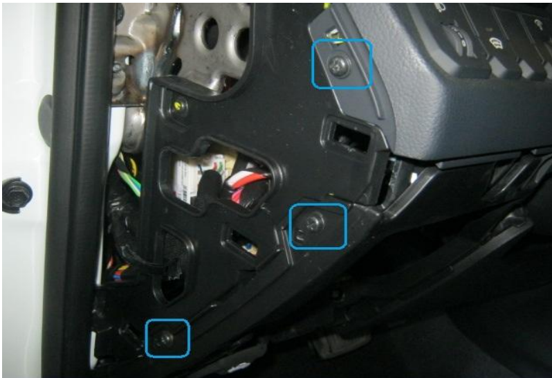
Фото 1.3. Крепление подторпедника
