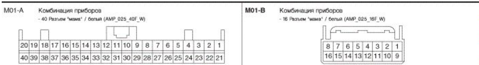
Фото 10. Разъемы приборного щитка.
