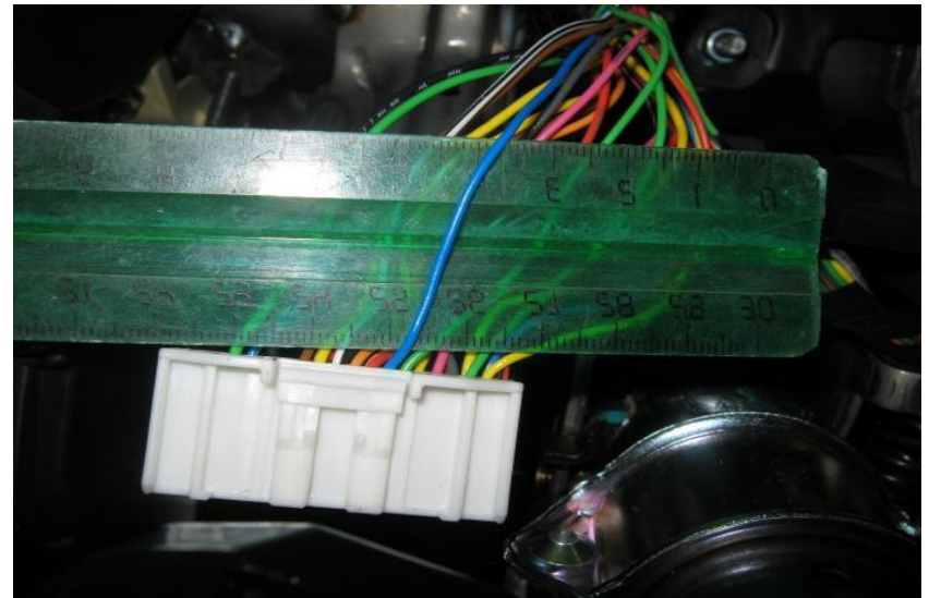
Фото 11.4. Генератор (Синий, №8 разъёма M01-A)
