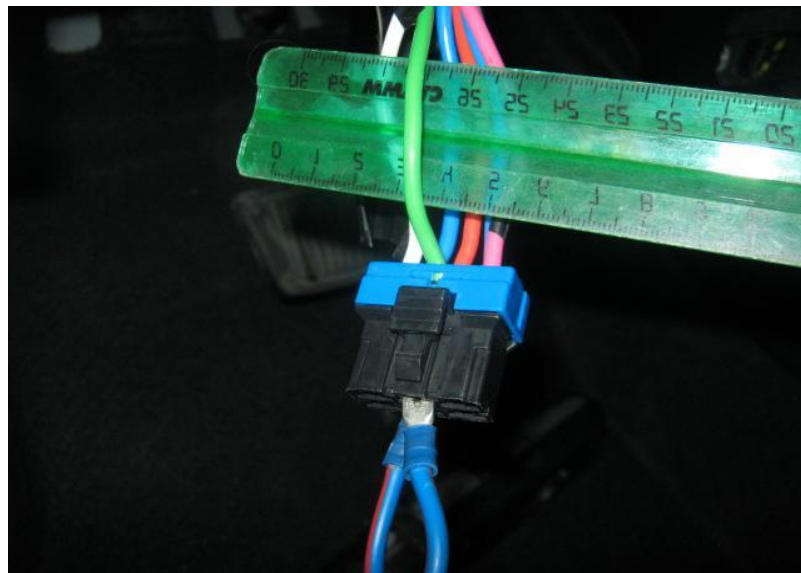
Фото 14.3. Зажигание 2 (Зелёный, № 2 разъёма M17)
