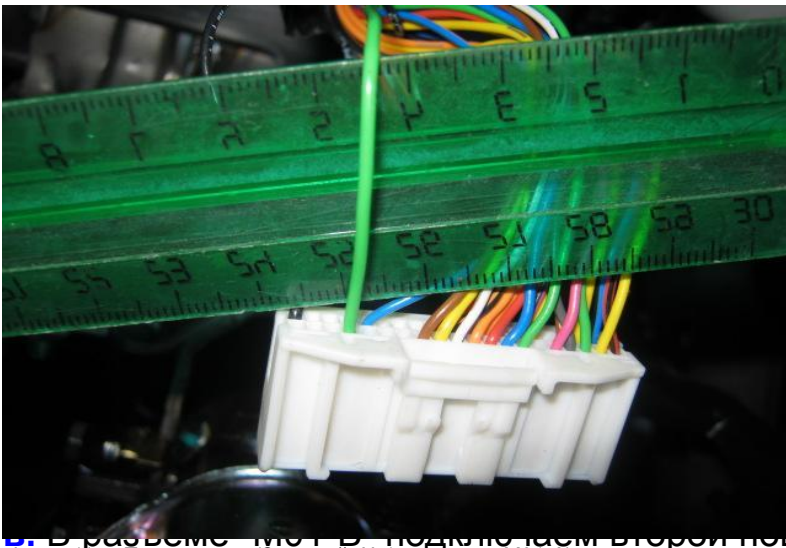
Фото 11.5. Поворотник (Зелёный, №17 разъёма M01-A)
