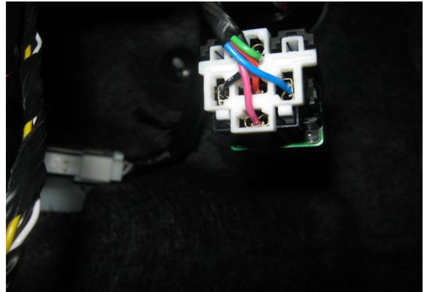
Фото 12.3. Тормоз (Розовый, №1 разъёма M32)
