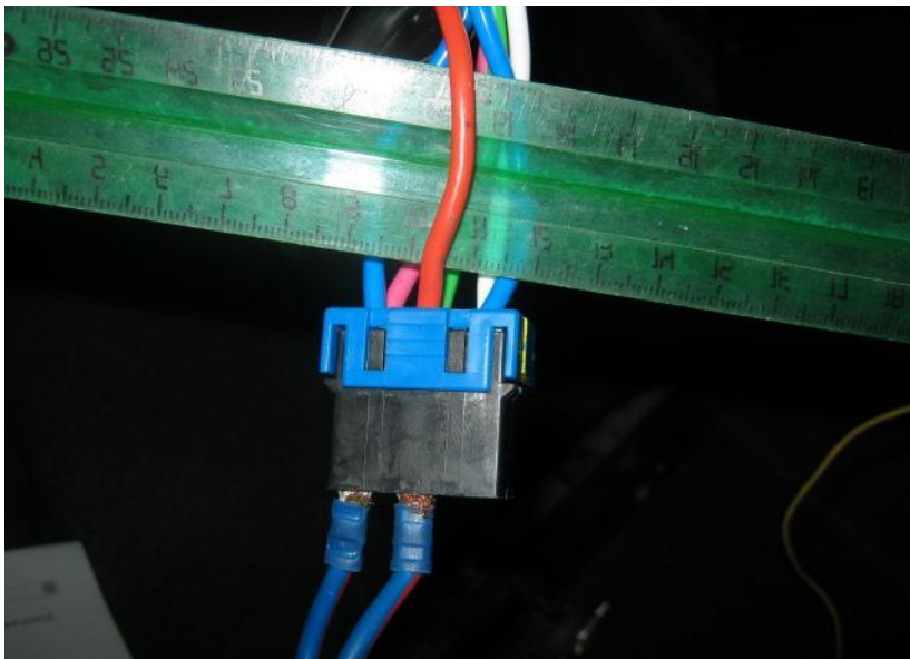
Фото 14.6. Постоянный плюс (Красный № 5 разъёма M17)
