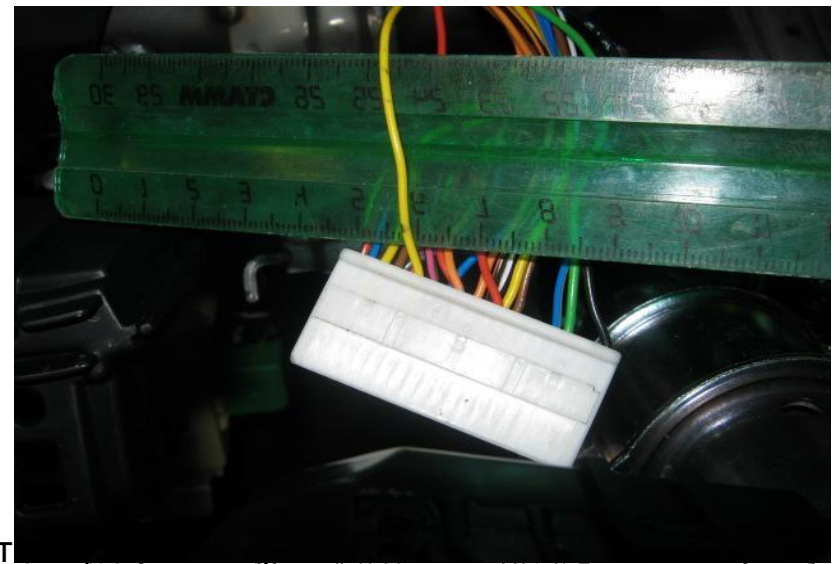
Фото 11.6. Зажигание (Жёлтый, №26 разъёма M01-A) Для питания модуля обхода
