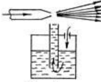
1. Схема распылителя
