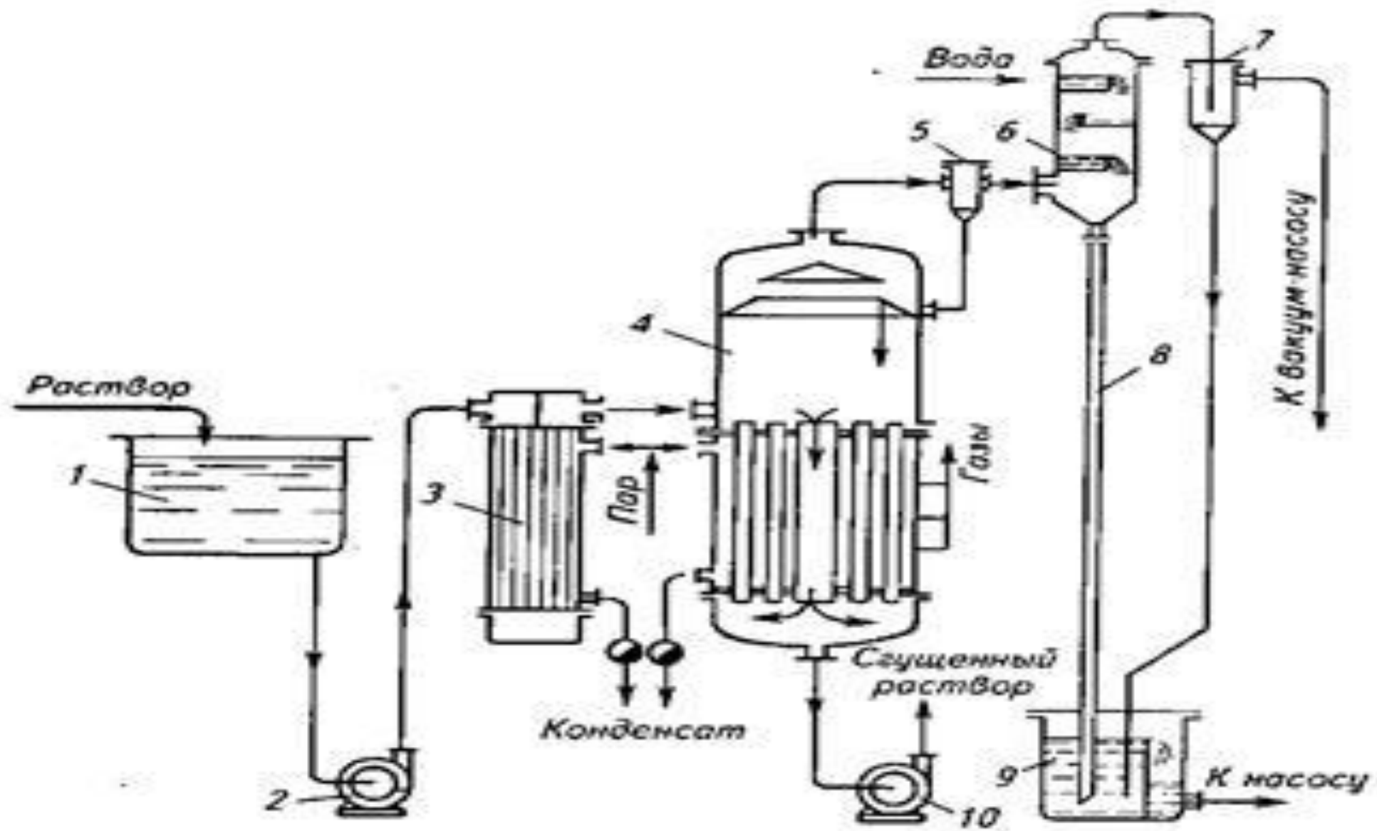
Рис. 26.2. Схема однокорпусной вакуумной выпарной установки
