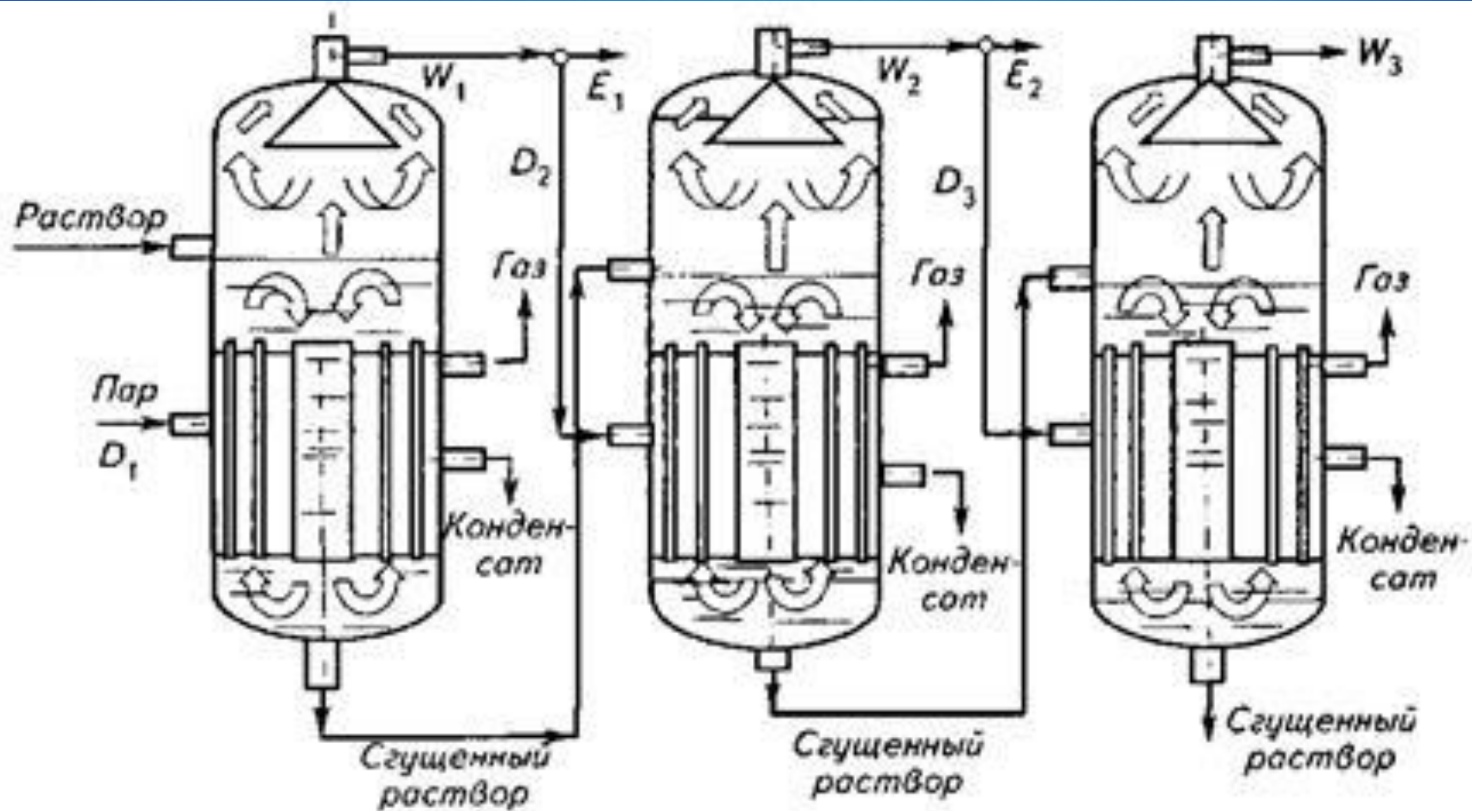
Рис. 26.3. Схема трехкорпусной вакуум-выпарной установки
