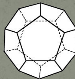
Додекаэдр {5,3}
