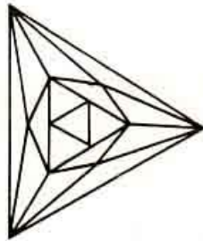
ИКОСАЭДР
