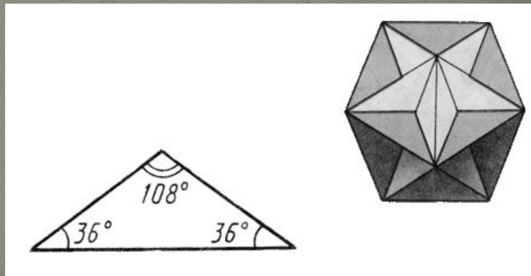
Большой додекаэдр
