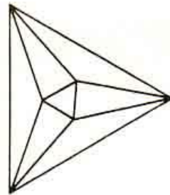
ОКТАЭДР
