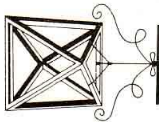
ОКТАЭДР
