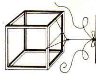
КУБ
