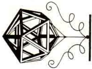
ИКОСАЭДР
