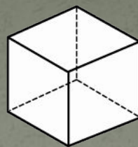
Куб {4,3}
