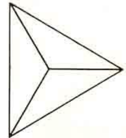
ТЕТРАЭДР
