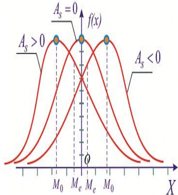
Асимметрия распределения
