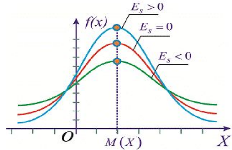
Эксцесс распределения
