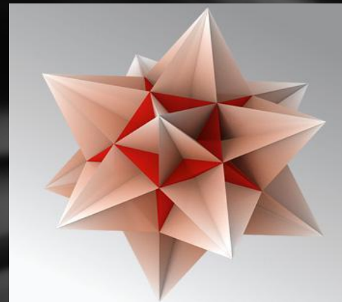
большой икосаэдр
