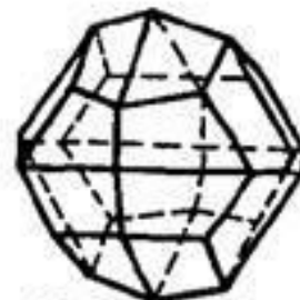
Дидодэкаэдр
