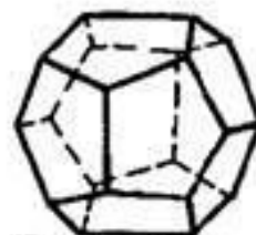
Пентагон- додэкаэдр
