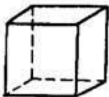
Гексаэдр
