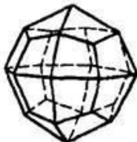
Тетрагон- триоктаэдр
