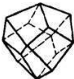
Тетрагон- тритетраэдр
