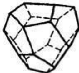
Пентагон- тритетраэдр
