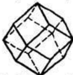
Ромбододекаэдр
