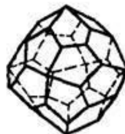
Пентагон- триоктаэдр
