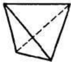
Тетраэдр
