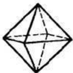
Октаэдр
