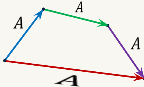
Правило многоугольника
