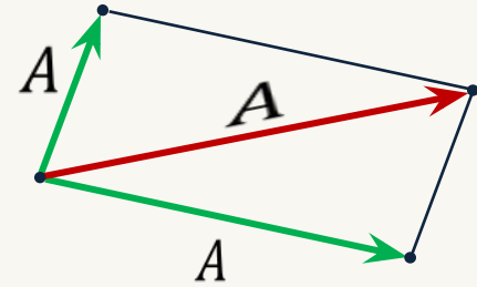
Правило параллелограмма
