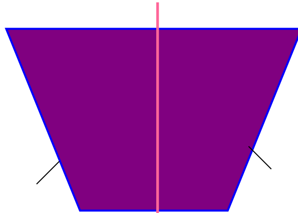
Равнобедренная трапеция
