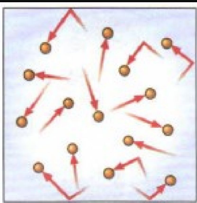
Хаотическое движение молекул газа
