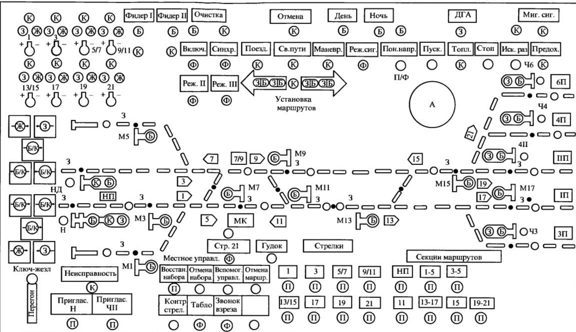
Лицевая панель пульта-табло
