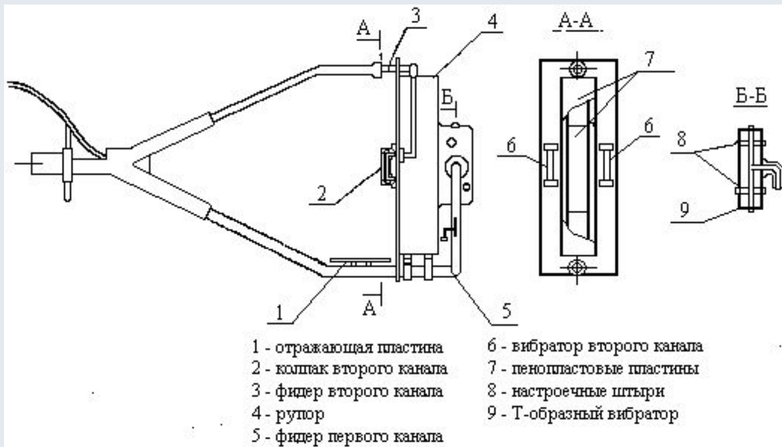
Рис. 3 Облучатель
