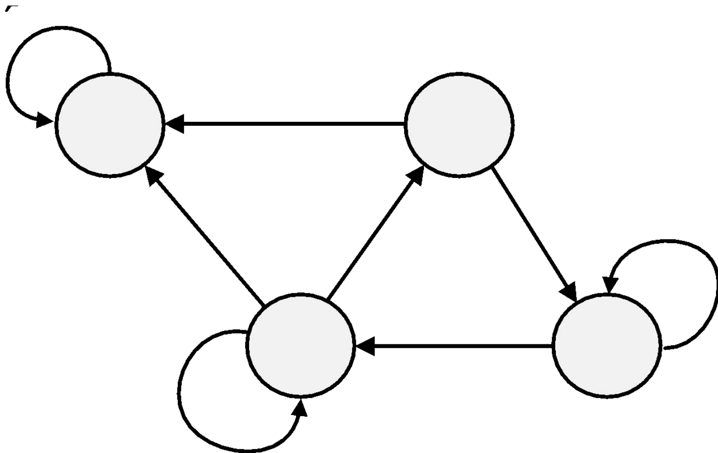
Матрица переходных вероятностей (P)
