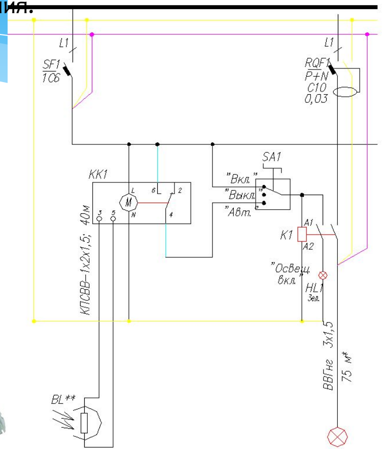
Фотореле ФРЛ-11
