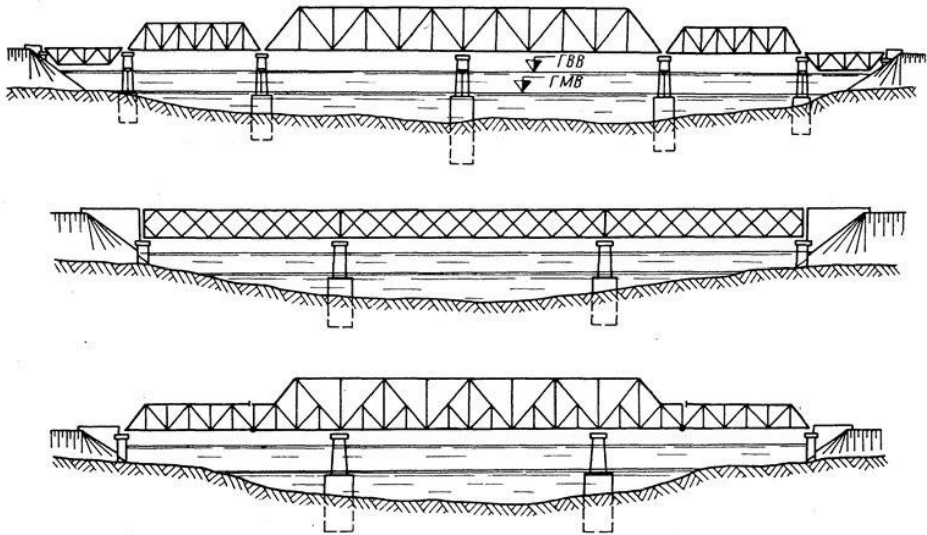
Рис. 95. Схемы мостов со сквозными фермами
