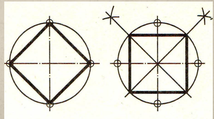
Деление окружности на 4 части
