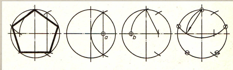
Деление окружности на 5 частей.
