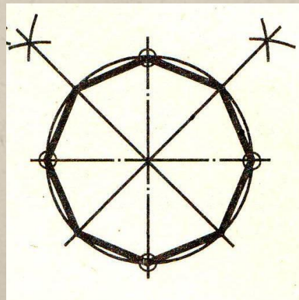
Деление окружности на 6 частей.
