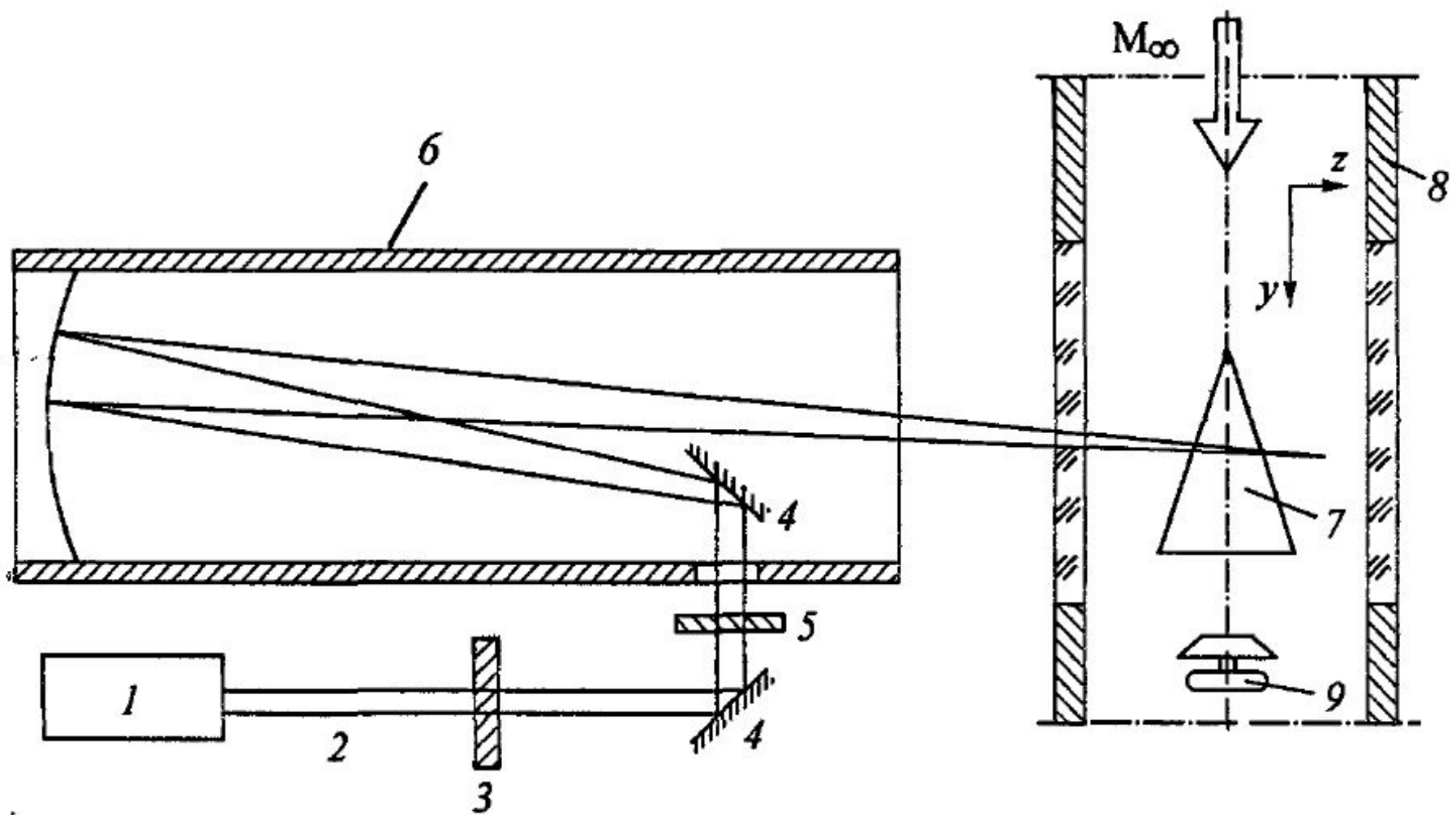
Оптическая схема формирования «лазерного ножа» [196]
