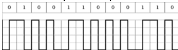
Дифференциальное манчестерское кодирование
