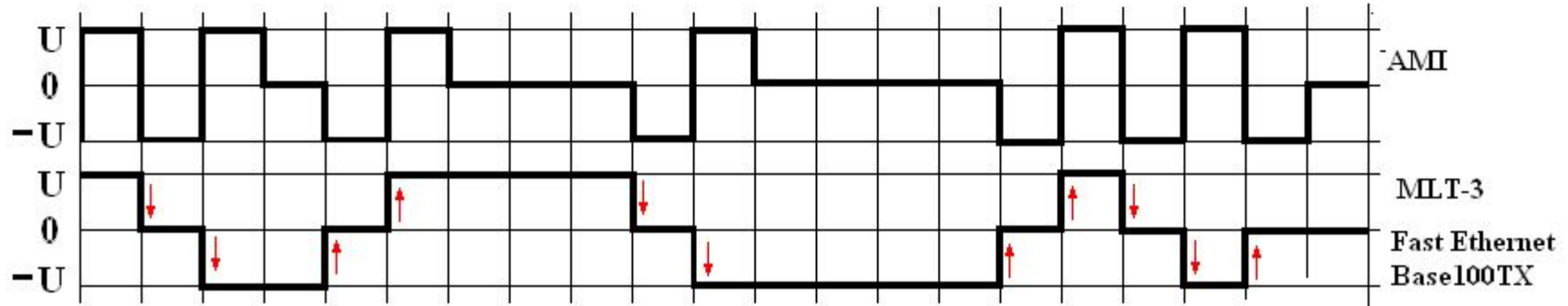
Тринарное кодирование Трехуровневый код
