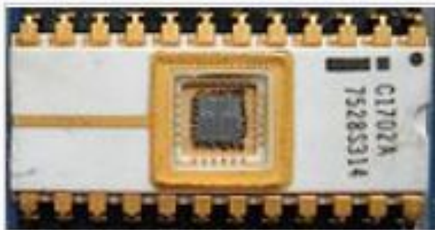
Микросхема EPROM Intel 1702 с ультрафиолетовым стиранием.
