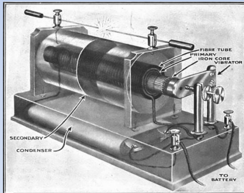
Конструкция индукционной катушки Румкорфа
