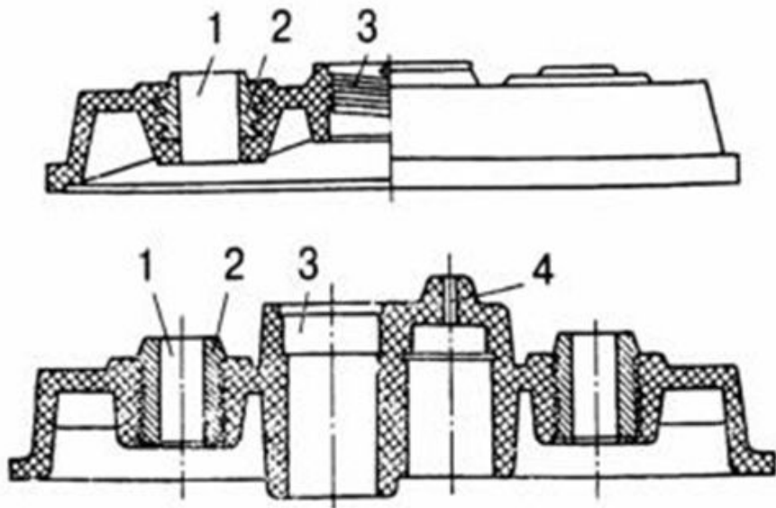
Рис. 8. Крышки для отдельной аккумуляторной ячейки моноблока:
