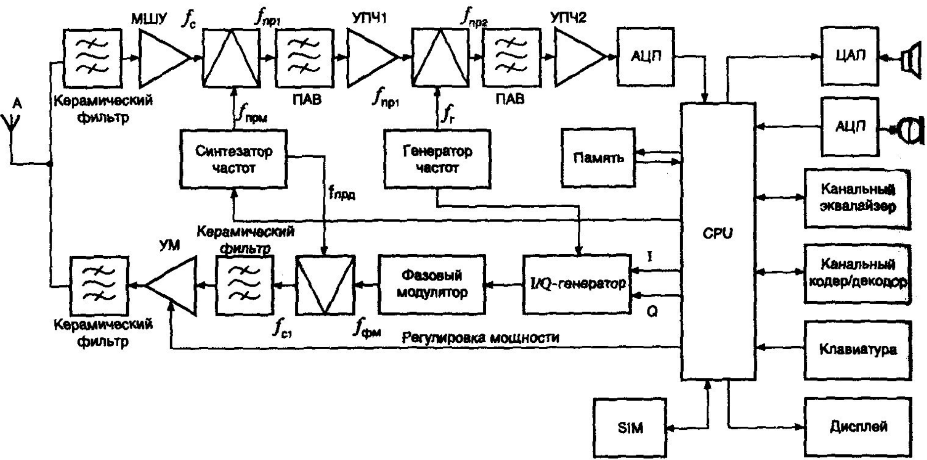
Структурная схема цифрового радиотелефона
