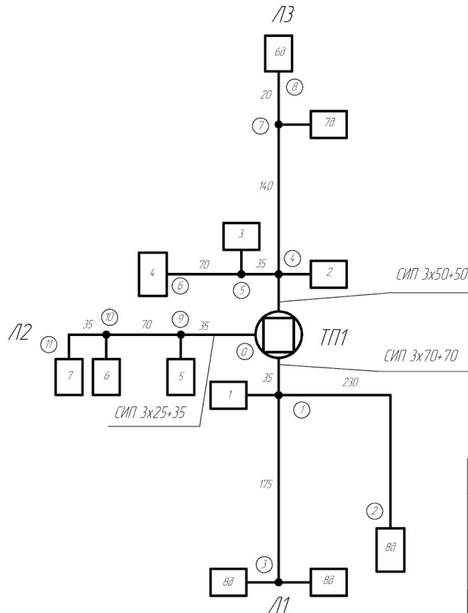
Мощность на участках ВЛ-0,38 кВ
