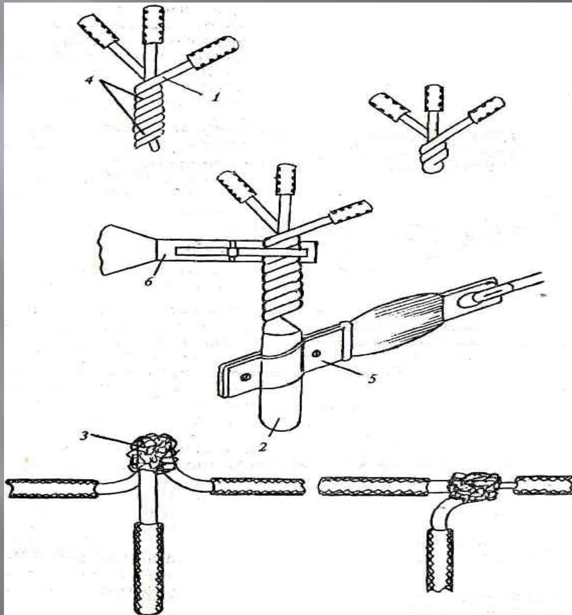
Рис. 139. Соединение проводов скруткой: 1 — отдельные жилы; 2 — электропровод (кабель); 3 — защитное покрытие скрутки; 4 — правильно выполненная скрутка; 5—6 — держатели проводов
