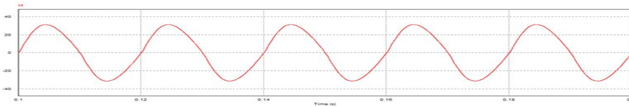
Ток на входе (а) и выходе (б) синус-фильтра
