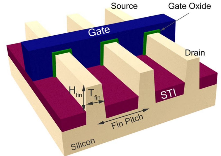
Плавниковый МОП-транзистор
