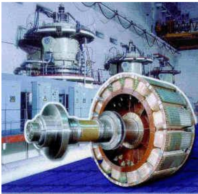
Явнополюсный ротор гидрогенератора с числом полюсов 16 ( p=8 )
