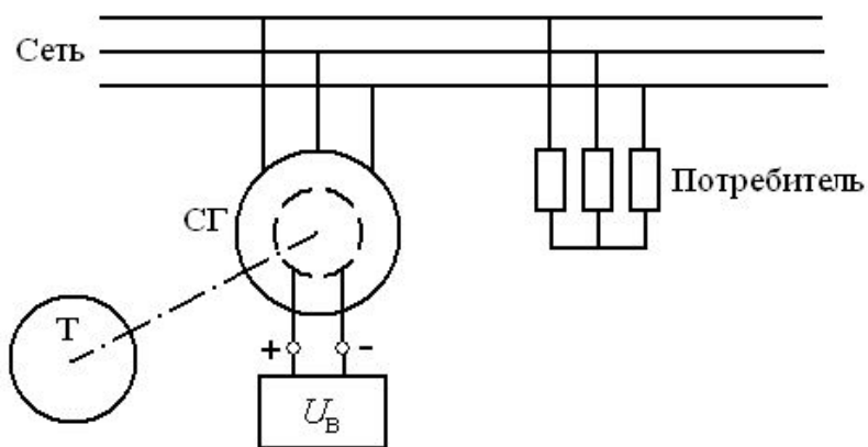
Схема включения синхронного генератора
