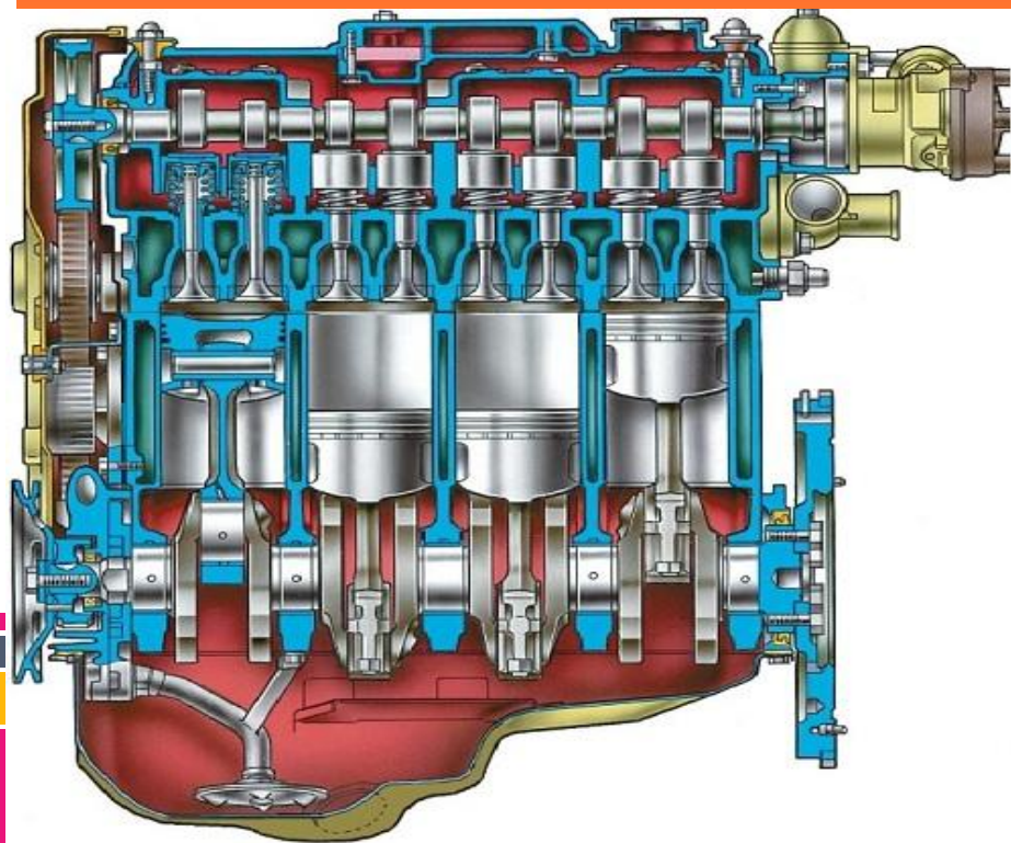
Бензиновый двигатель (карбюраторный)
