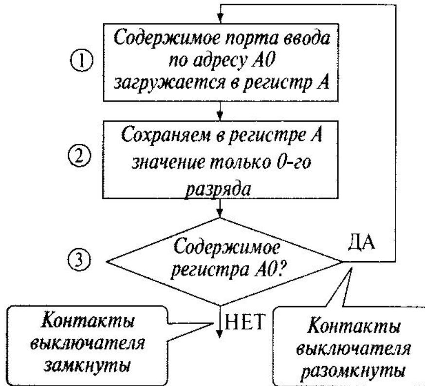
Схема алгоритма
