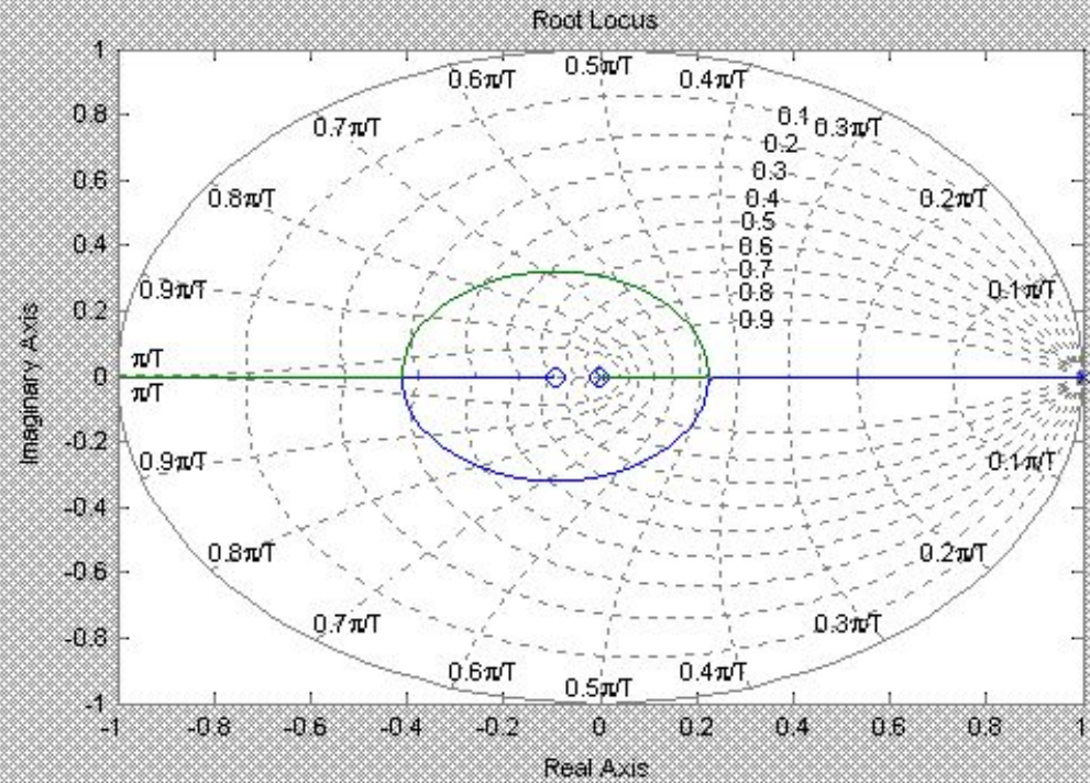
Корневой годограф для дискретной системы
