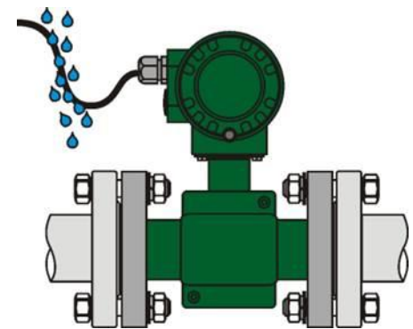
Кабель должен иметь U-петлю и дренажное отверстие (при применении гофрошланга)
