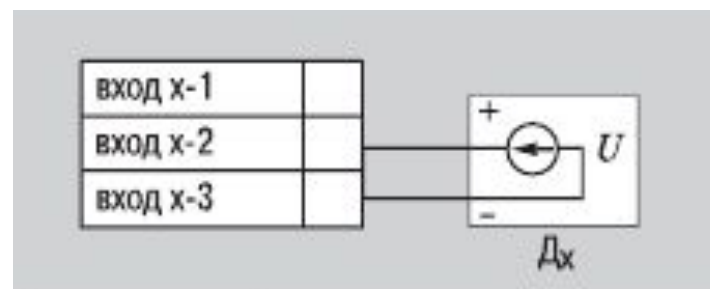
Датчик с унифицированным выходным сигналом напряжения
