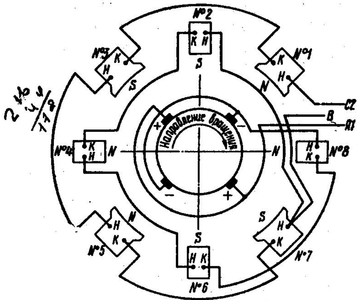
Рис. 44. Схема соединения катушек полюсов электродвигателя НБ-431П
