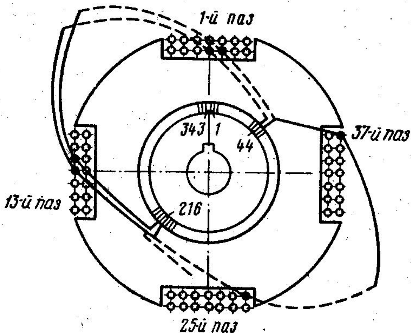
Рис. 45. Схема соединения обмотки якоря электродвигателя НБ-431П
