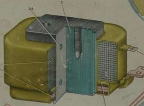
ДОБАВОЧНЫЙ ПОЛЮС
