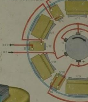
СХЕМА СОЕДИНЕНИЯ КАТУШЕК ДОБАВОЧНОГО ГЕНЕРАТОРА ПРЕОБРАЗОВАТЕЛЯ
