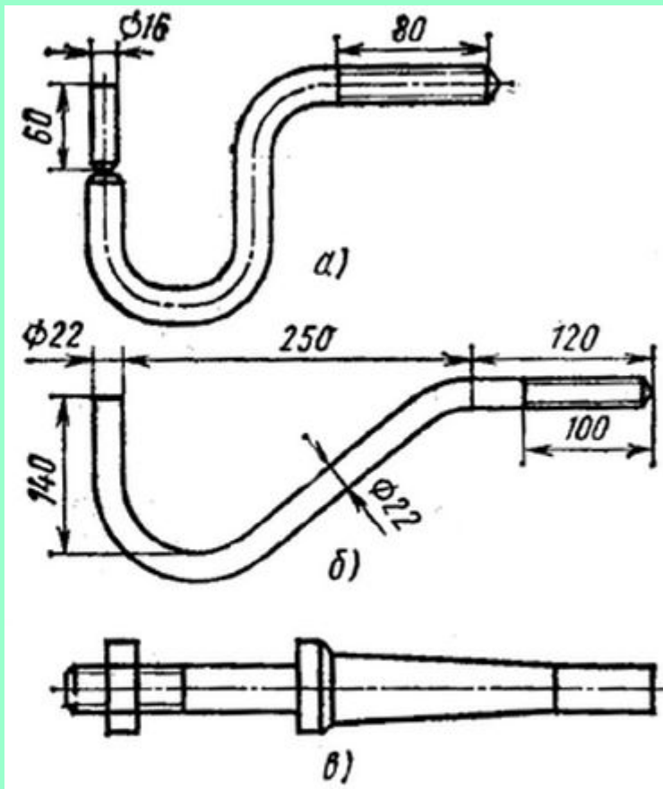
а - крюк КН-16, б - крюк КВ-22, в - штырь ШН
