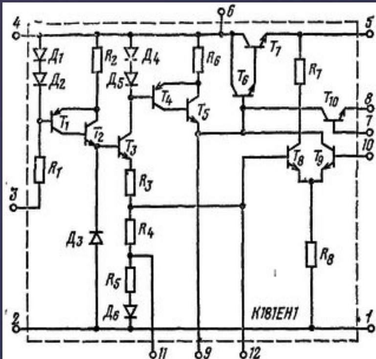
Рис. 2.28. Микросхема К181ЕН1
