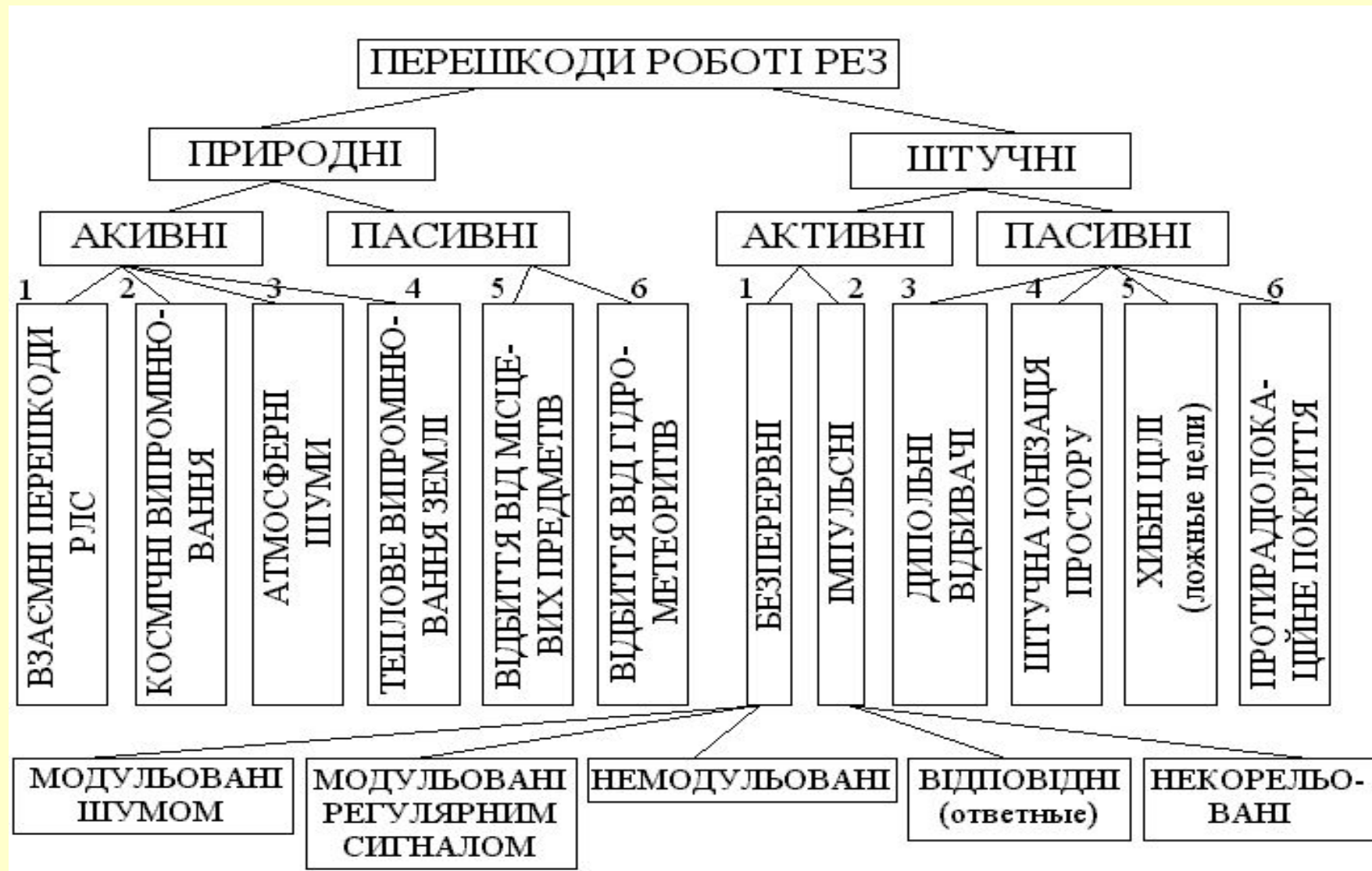
Рис.1. Класифікація перешкод
