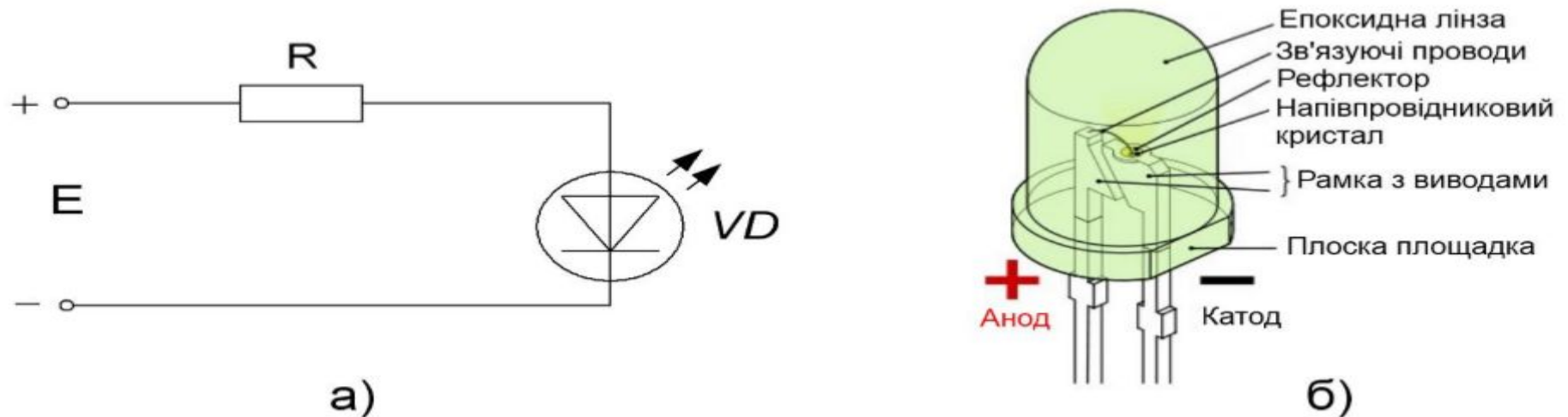
Рис.2.20. Схема ввімкнення (а) та будова світлодіода (б)
