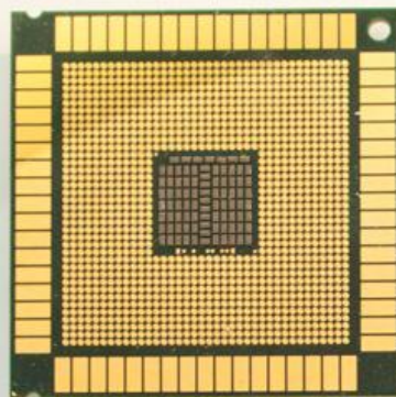
Серверный процессор Intel® Itanium® с терморассеивателем
