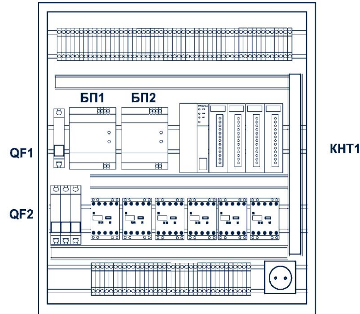
Шкаф автоматизации
