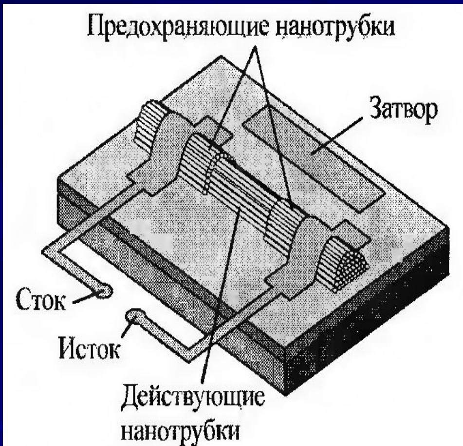
Рис. 1.16. Схема нанотранзистора на углеродной нанотрубке
