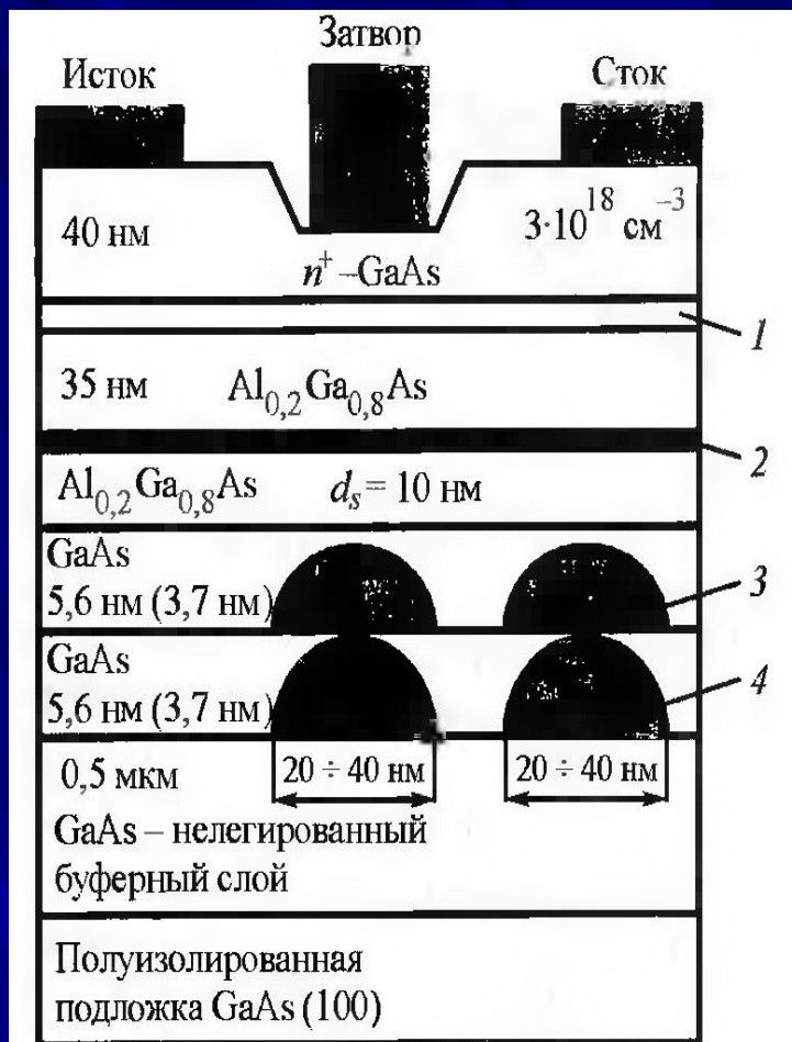
Рис. 1.14. Структура модулированно-легированного транзистора с квантовыми точками: 1 — нелегированный слой GaAs (6 нм); 2 — \delta(\text{Si}) -слой ( 2 \cdot 10^{12} \text{ см}^{-2} ); 3, 4 — InAs 1,07 нм (0,7 нм)
