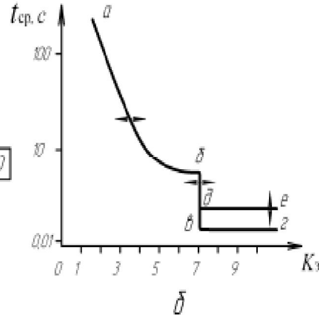
Структурная схема электронного расцепителя ( а ) и его защитная характеристика ( б ): 1, 2, 3 – датчики тока; 4 – блок преобразования; 5, 8 – блоки контроля уровня сигнала; 6, 9 – блоки временной задержки; 7 – усилитель или компаратор; 10 – исполнительный орган
