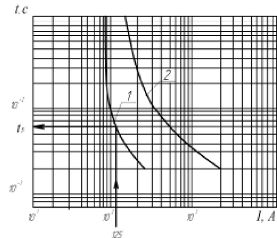
Рисунок 2.6 – Времятоковые характеристики быстродействующего предохранителя ПП50 на номинальный ток плавкой вставки 25 А: 1 – преддуговой время; 2 – полное время срабатывания
