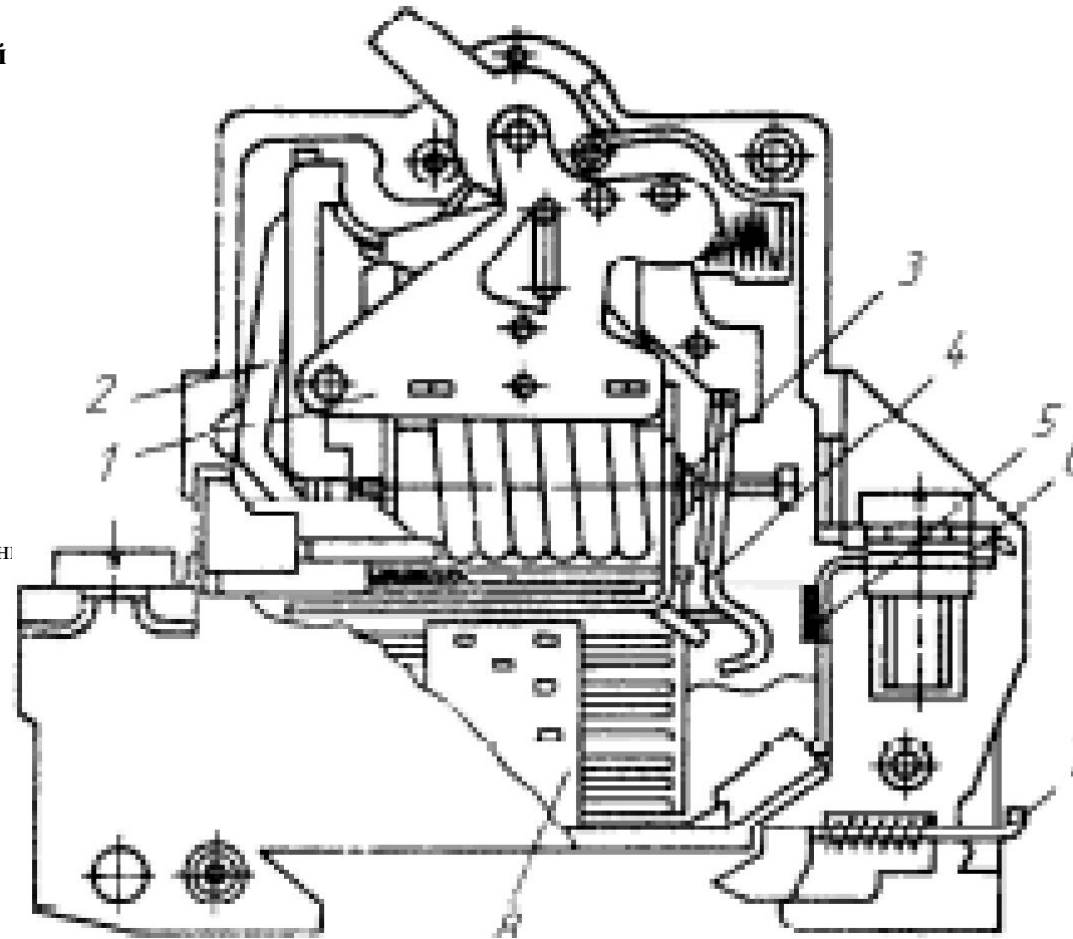
Однополюсный автоматический выключатель ВА14:
