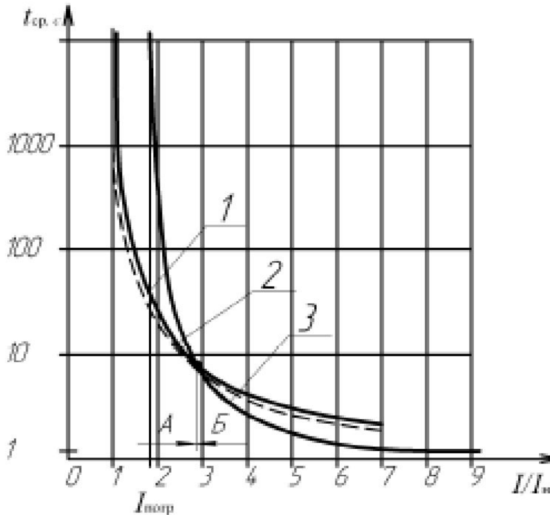
Рисунок 2.1 – Времятоковые характеристики 1 – электрооборудования; 2 – идеального предохранителя; 3 – реального предохранителя
