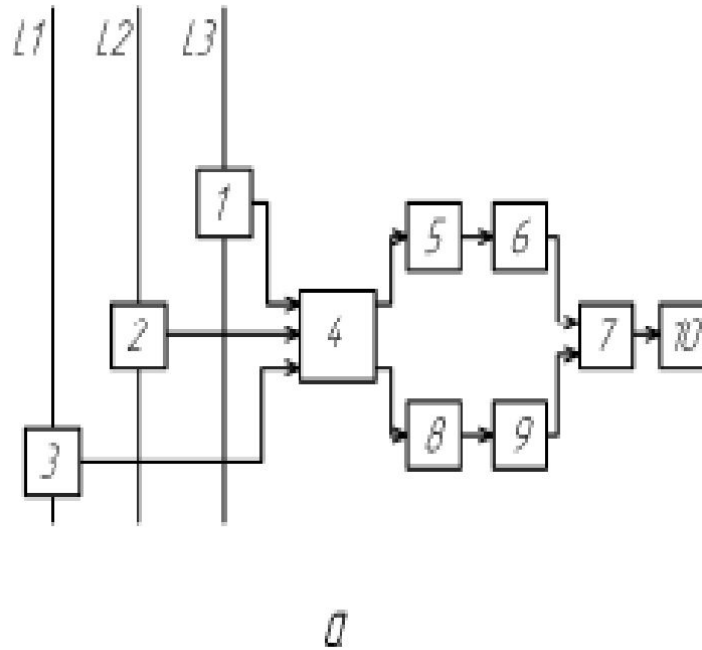
Структурная схема электронного расцепителя ( а ) и его защитная характеристика ( б ): 1, 2, 3 – датчики тока; 4 – блок преобразования; 5, 8 – блоки контроля уровня сигнала; 6, 9 – блоки временной задержки; 7 – усилитель или компаратор; 10 – исполнительный орган
