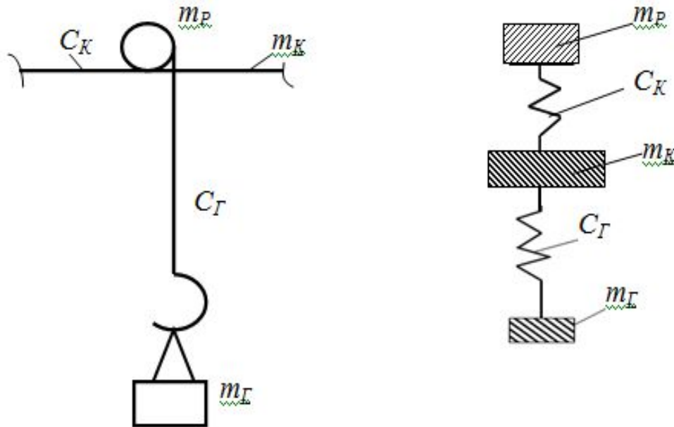
Расчетная схема мостового крана с грузом
