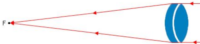
Объектив-рефрактор ахроматический
