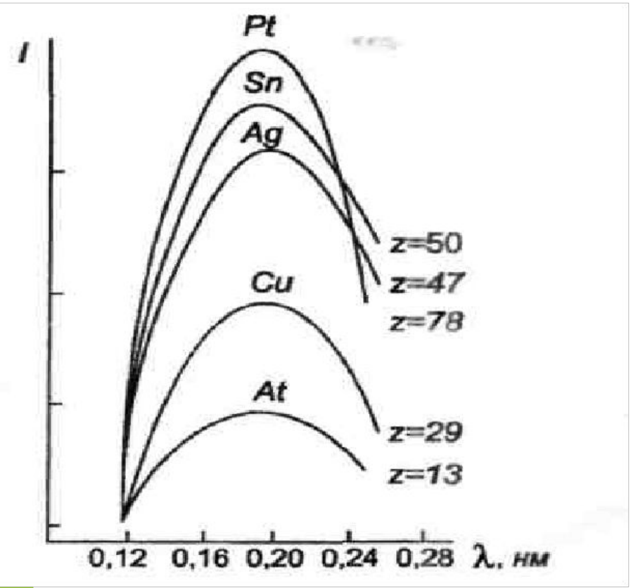
1.2сурет. Тежеуішті үздіксіз спектрлердің толқын ұзындығына тәуелділік түрі
