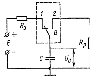
Схема генератора развертки
