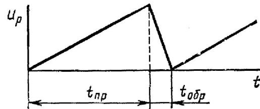
Развертывающее напряжение осциллографа
