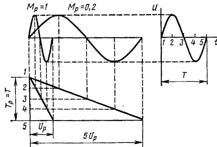
Изображение исследуемого сигнала при M_p = 1 ; M_p = 0,2
